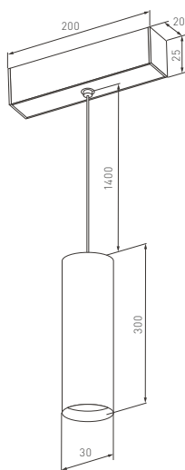
Рис. 1. Чертеж и габаритные размеры
