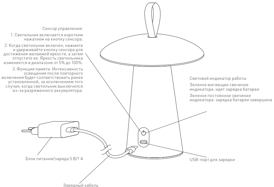
Рис. 2. Подключение светильника
