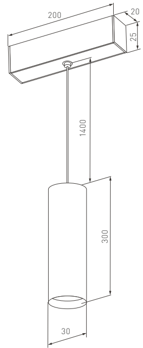
Рис. 1. Чертеж и габаритные размеры
