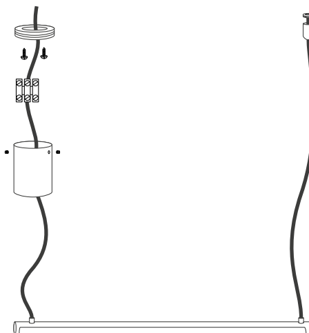
Рис. 2. Установка и подключение светильника
